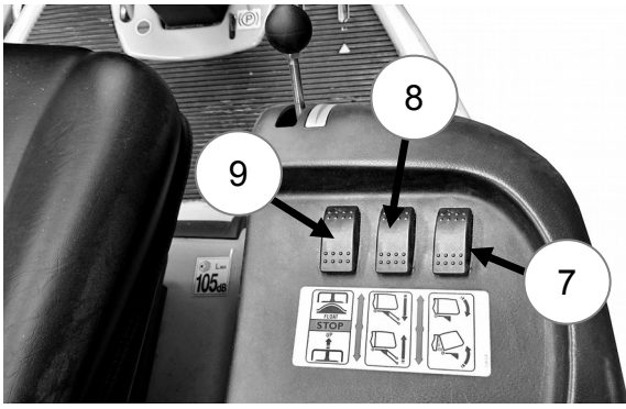
FIG. 1 – COMMANDS FIG. 1 – COMANDI FIG. 1 – COMMANDES ABB. 1 – BEDIENUNGEN FIG. 1 – COMANDOS
